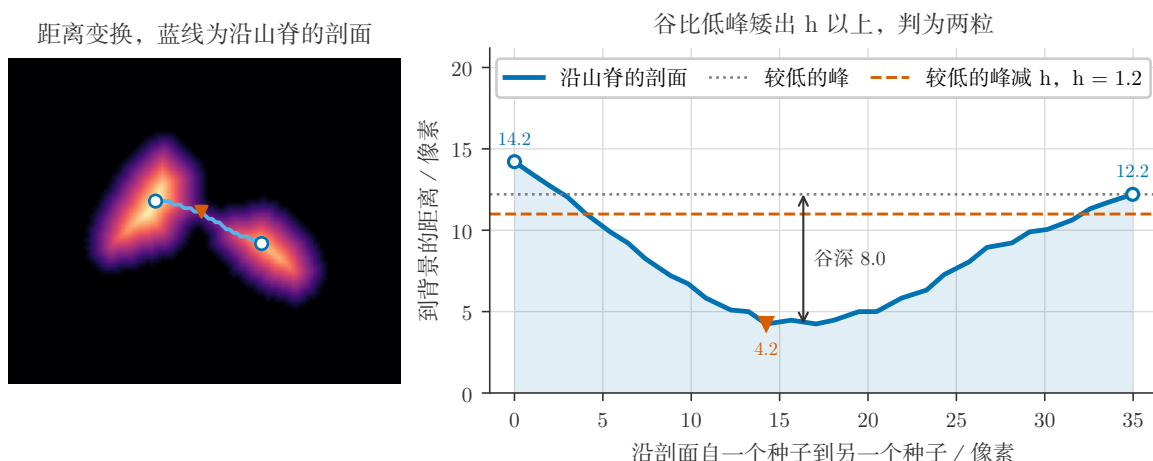
图 8: 为什么看深度而不看距离。左为粘连块的距离变换，右为沿山脊的剖面。谷底低于红色虚线，即比较低的峰矮出 h 以上，两个峰各留一个种子。
