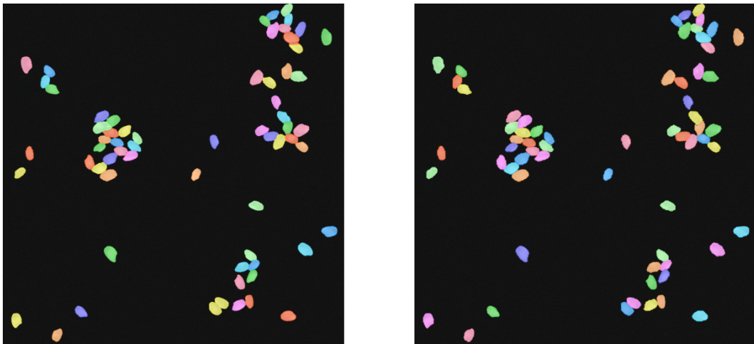
图 14: 合成粘连图 D2 中重度粘连场景的结果, 左为本文方法、右为 SAM 3。
