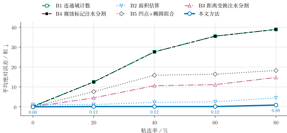
图 11: 计数误差随粘连率的变化。
