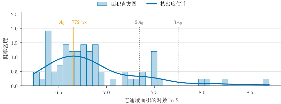
图 6: 面积分布的最高峰即单粒面积 A_0 , 粘连块集中在它的整数倍附近。
