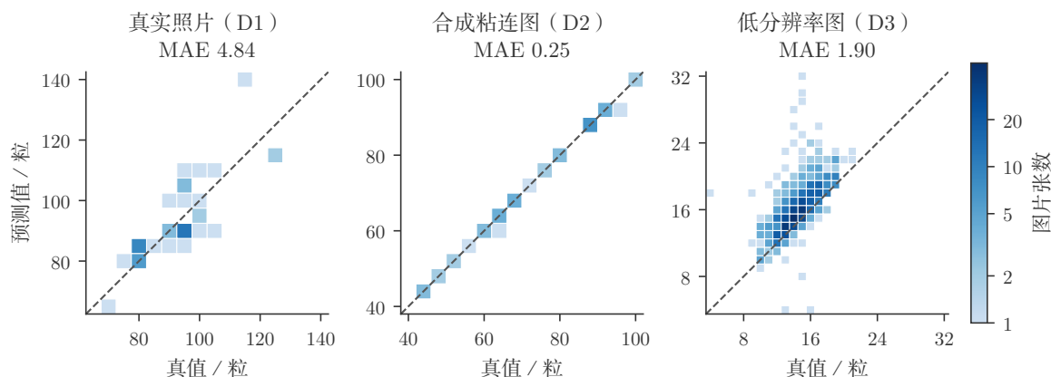
图 12: 预测值与真值对照的热力图。格子颜色表示落在该格的图片张数，虚线表示两者相等。
