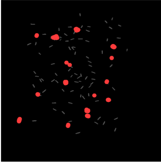
图 10: B3 的全局阈值与本文自适应种子的对照, 红色为种子, 灰色为二值图。本文对每个连通域分别放种子, 粘连块会得到不止一个, 因此总数多于米粒数。
