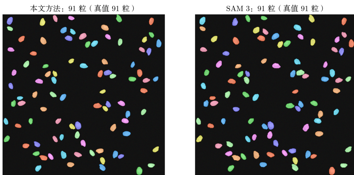
图 22: 合成粘连图 D2 中不粘连的场景，左为本文方法、右为 SAM 3。
