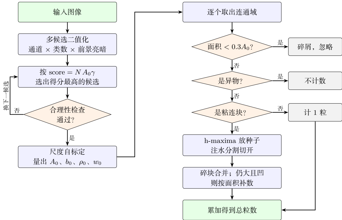
图 3: 方法流程图。
