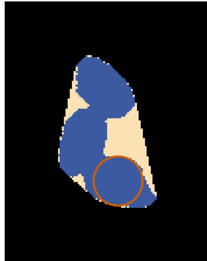
图 7: 单粒与粘连块的对照。蓝色为区域本身, 浅色为凸包多出的部分, 橙圈为最大内切圆。
