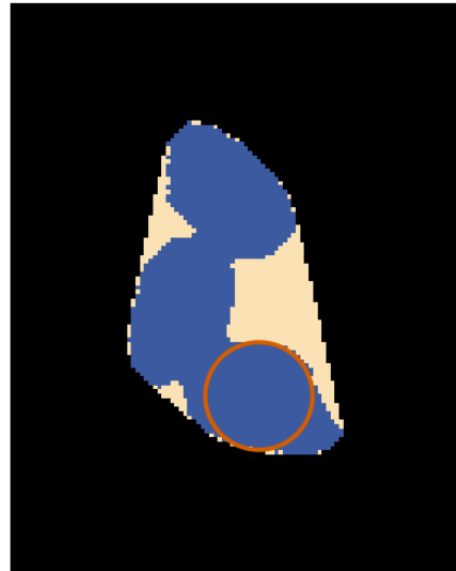
图 7: 单粒与粘连块的对照。蓝色为区域本身, 浅色为凸包多出的部分, 橙圈为最大内切圆。
