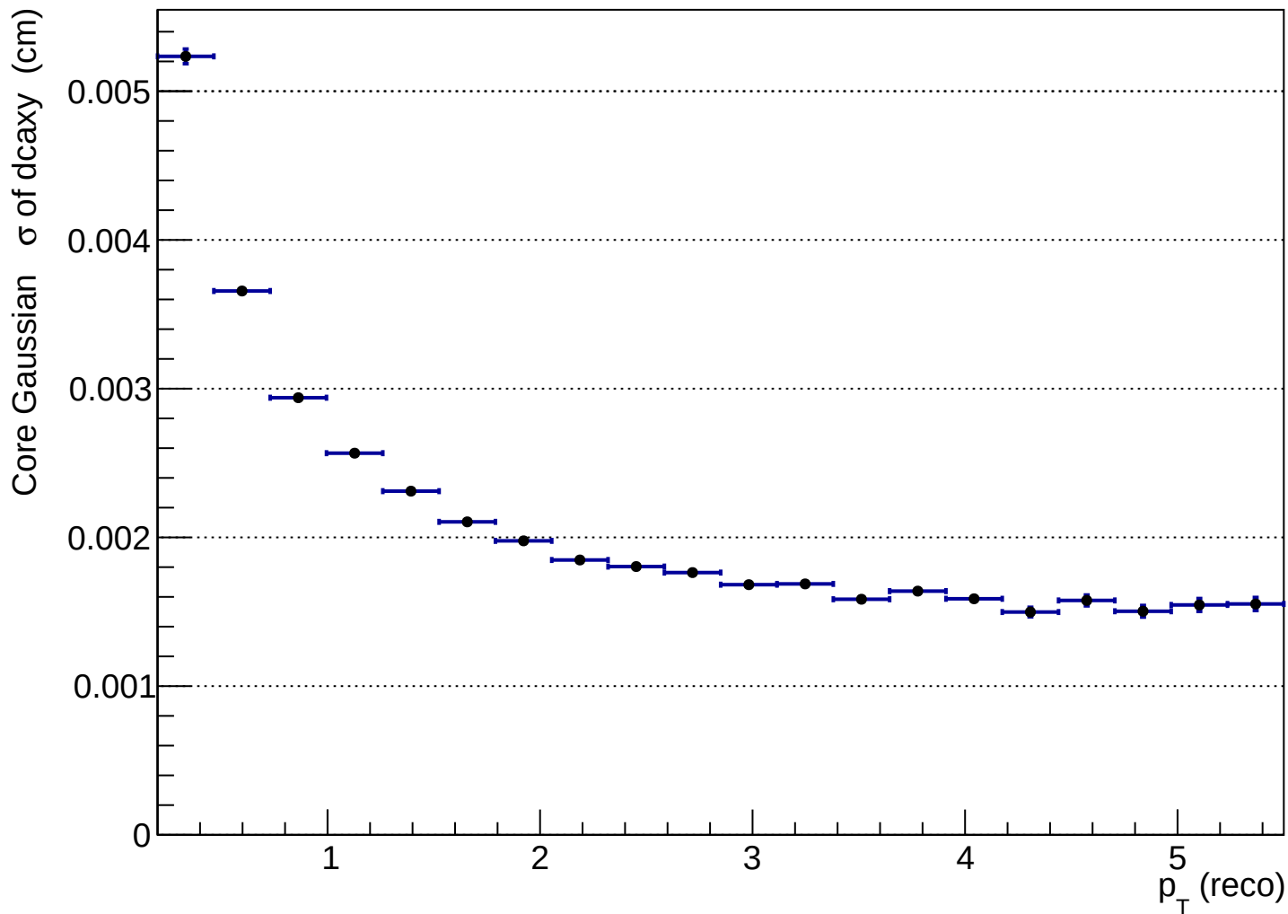
hdcaxy_vs_ptreco
