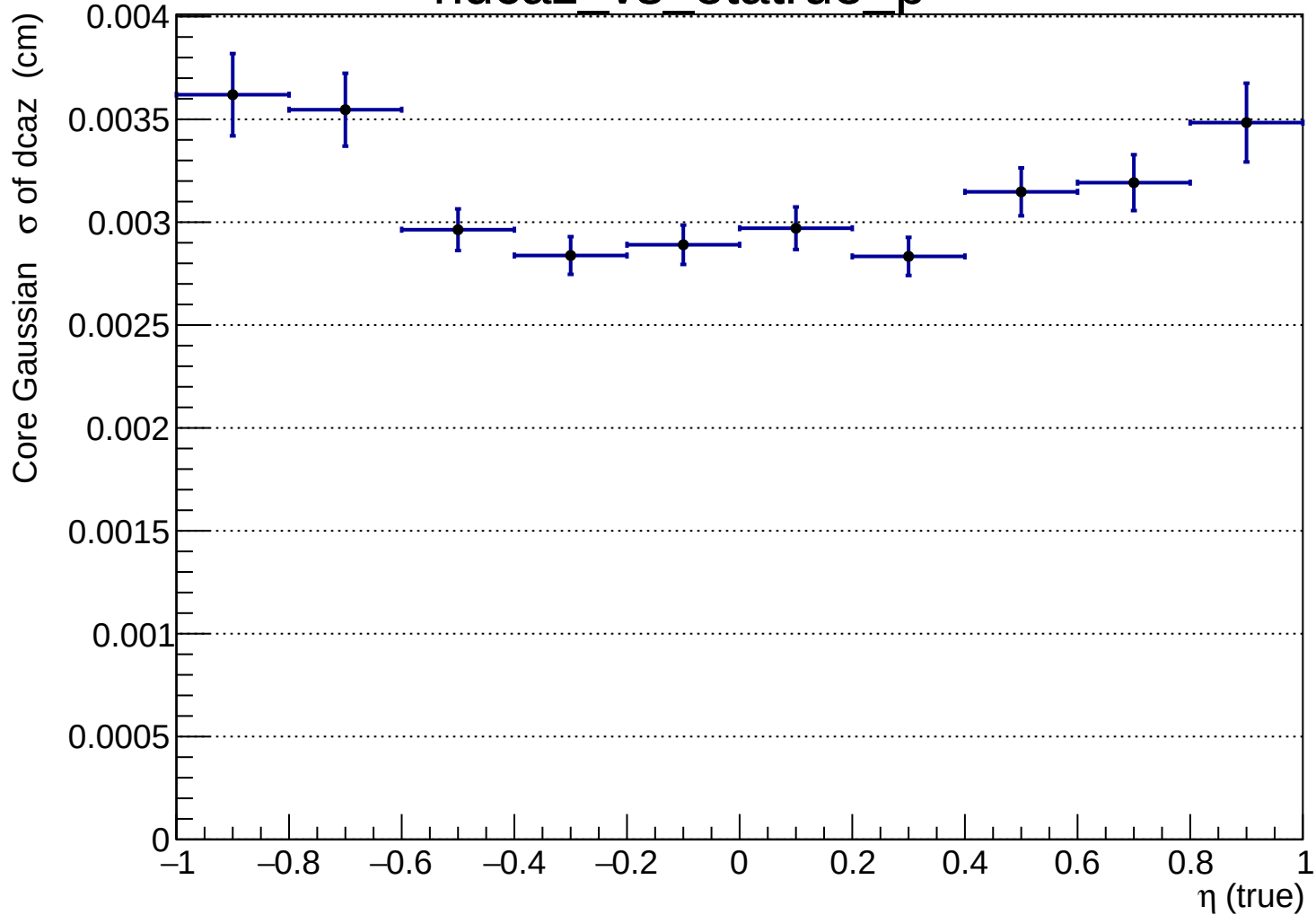
hdcaz_vs_eta_true_p
