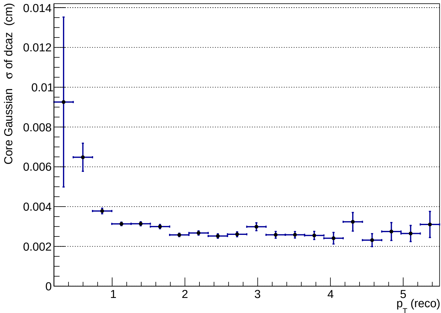
hdcaz_vs_ptreco_p
