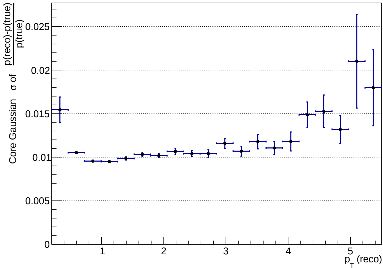
hpRes_vs_ptreco_K-
