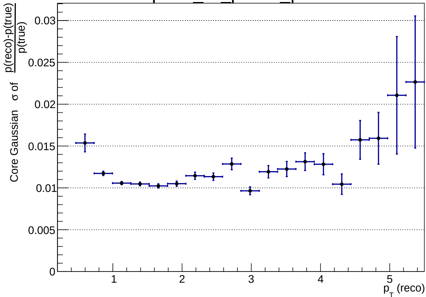
hpRes_vs_ptreco_p̄
