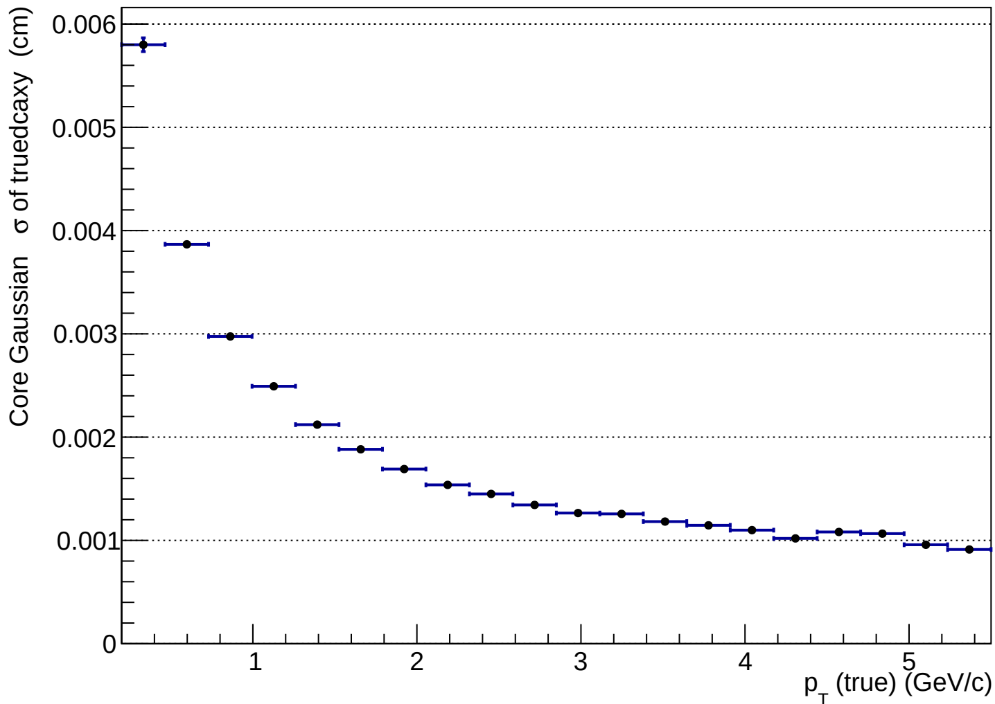
htruedcaxy_vs_pttrue
