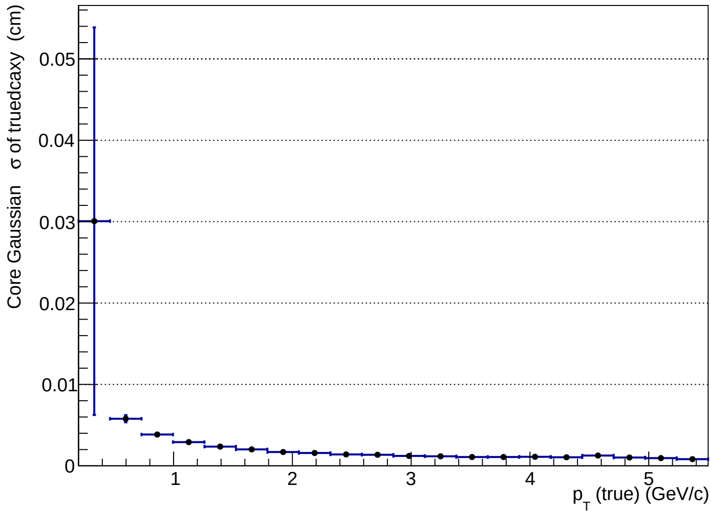
htruedcaxy_vs_pttrue_p
