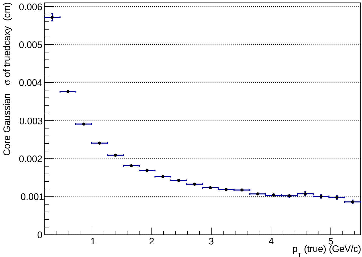
htruedcaxy_vs_pttrue_pi-
