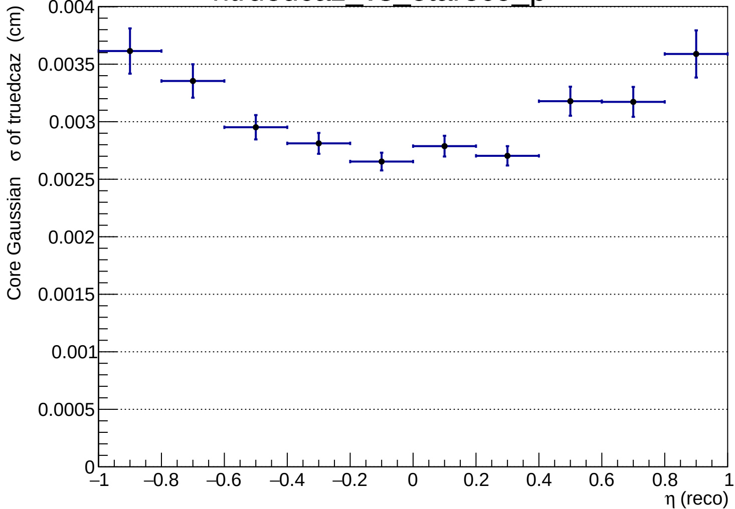
htruedcaz_vs_eta_reco_p̄
