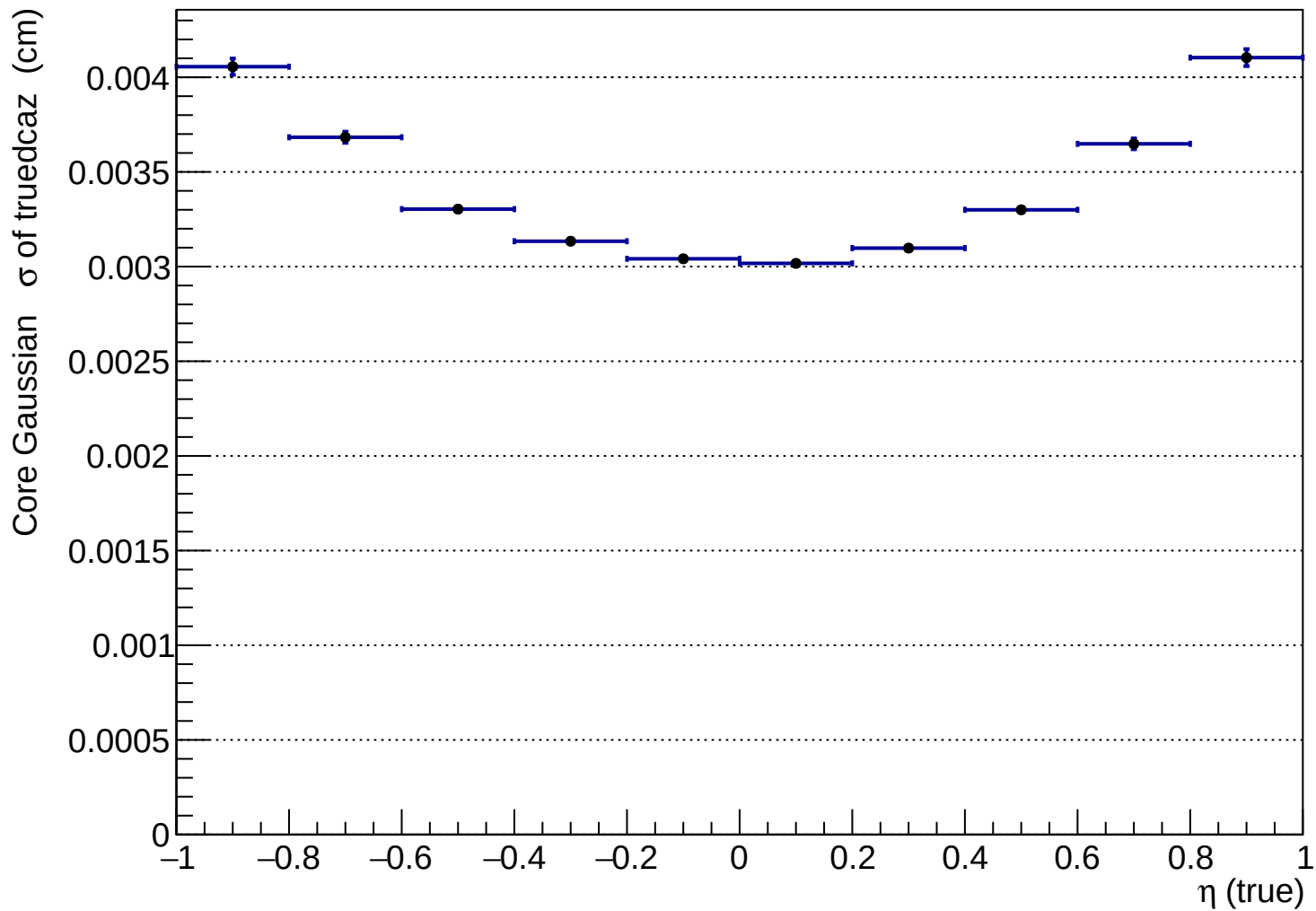
htruedcaz_vs_etatru
