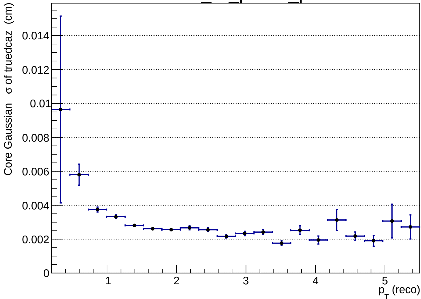
htruedcaz_vs_ptreco_p̄
