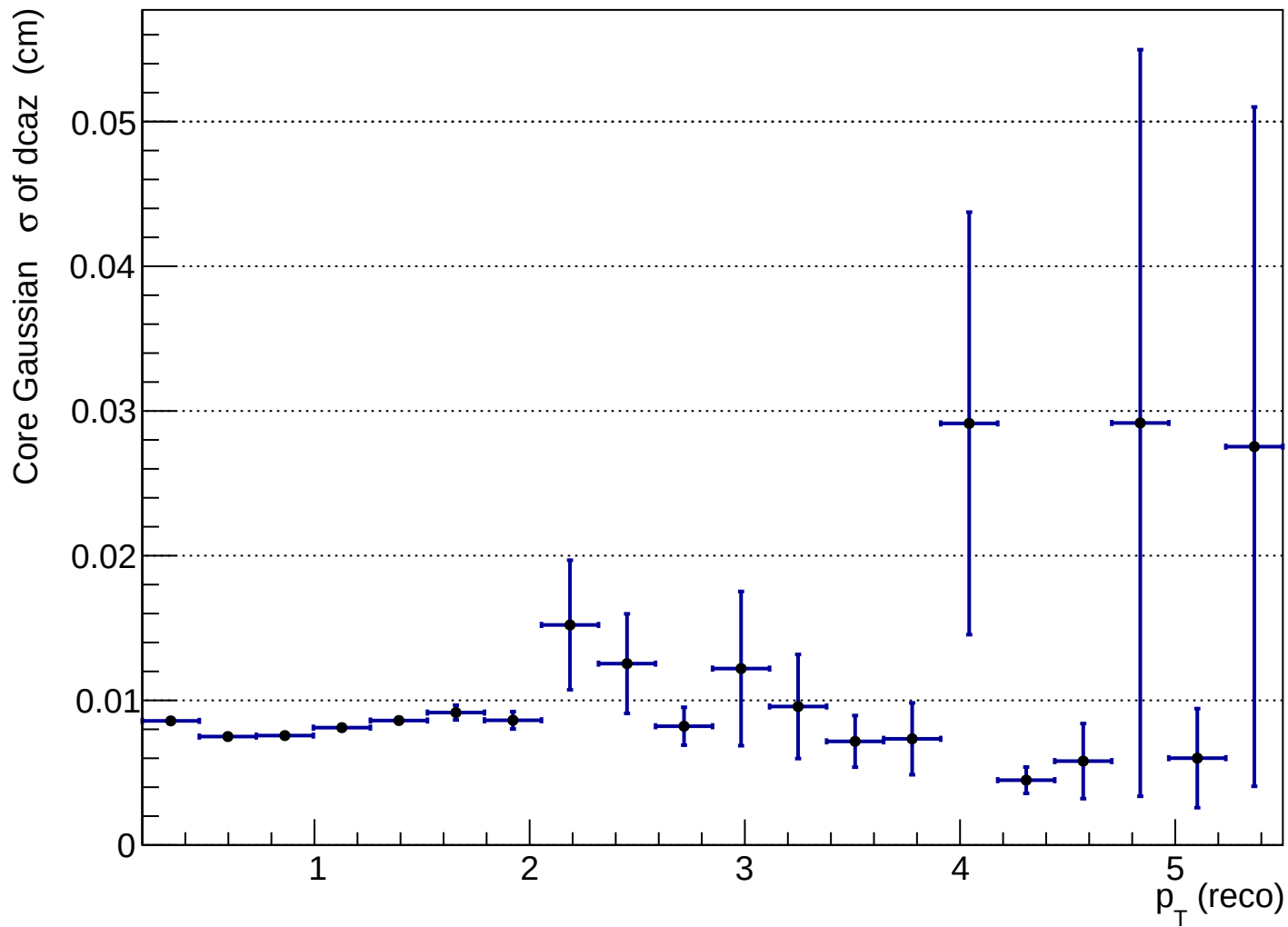
hdcaz_vs_ptreco
