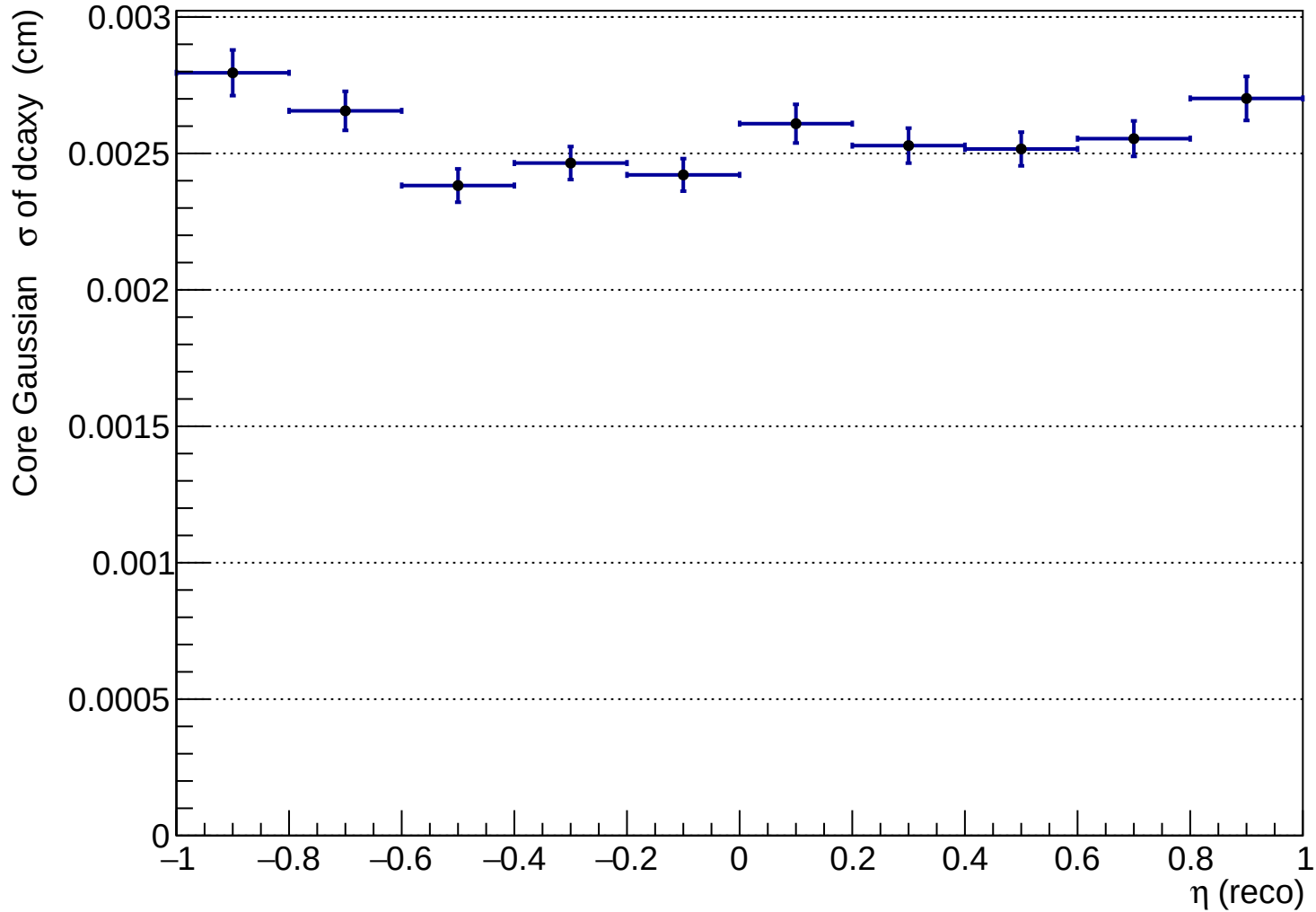
hdcaxy_vs_eta_reco_p
