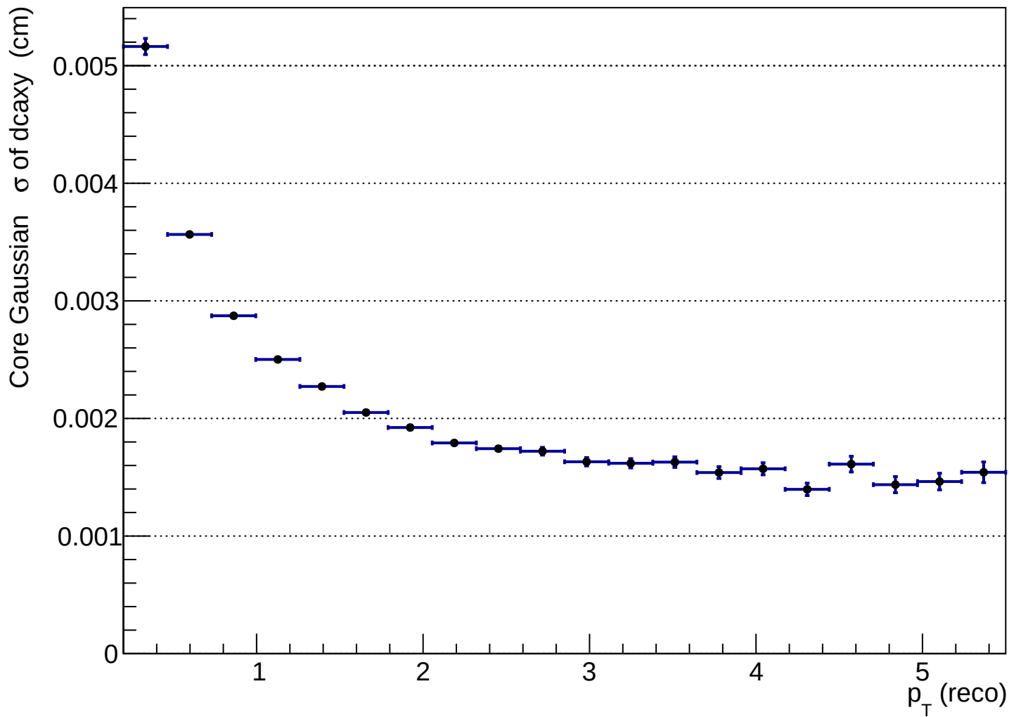
hdcaxy_vs_ptreco_pi-
