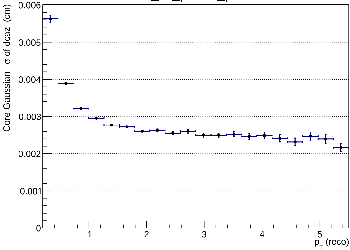
hdcaz_vs_ptreco_pi+
