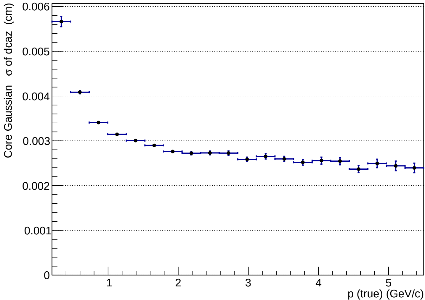
hdcaz_vs_ptrue_pi+
