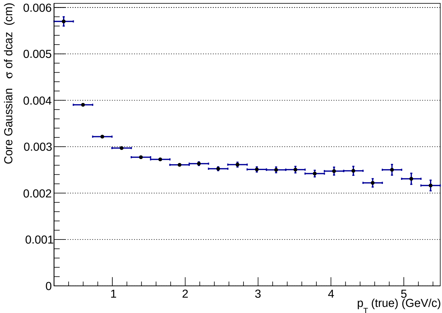
hdcaz_vs_pttrue_pi+
