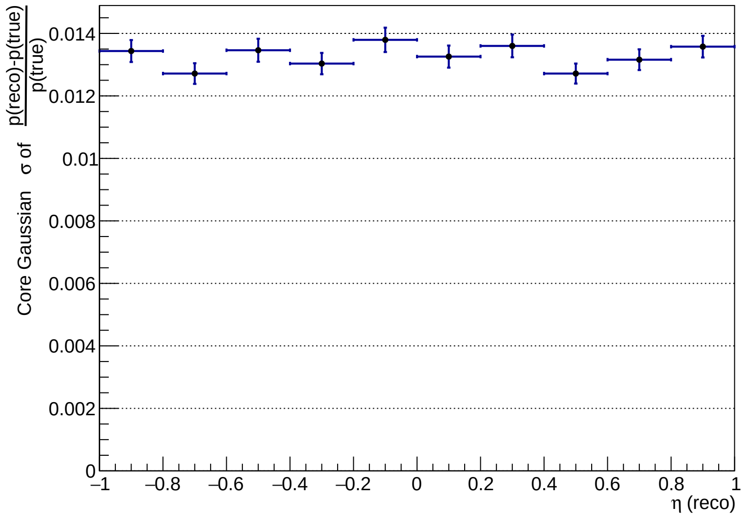
hpRes_vs_eta reco_p
