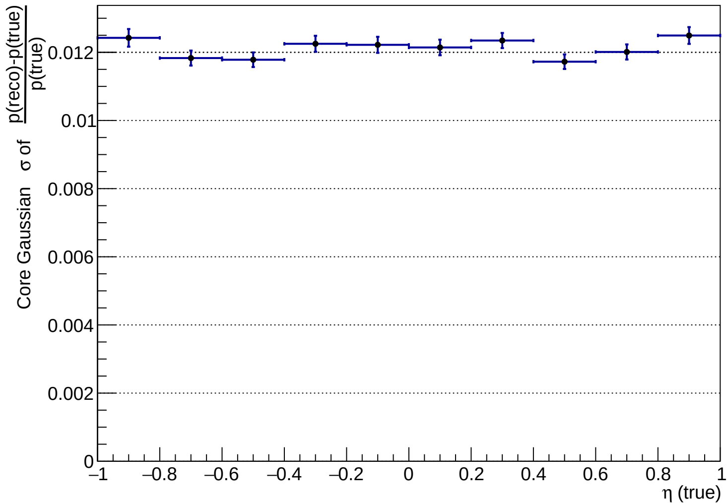
hpRes_vs_eta_true_K-
