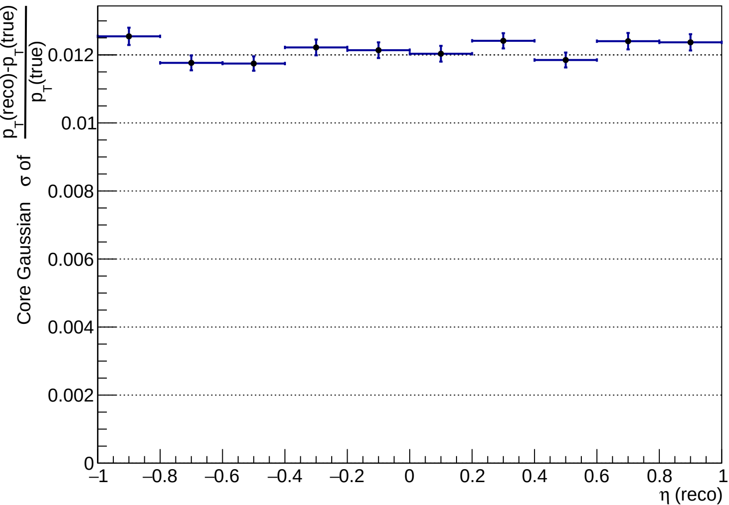
hptRes_vs_eta reco_K-
