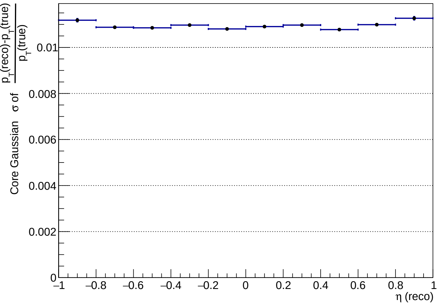
hptRes_vs_eta reco_pi-
