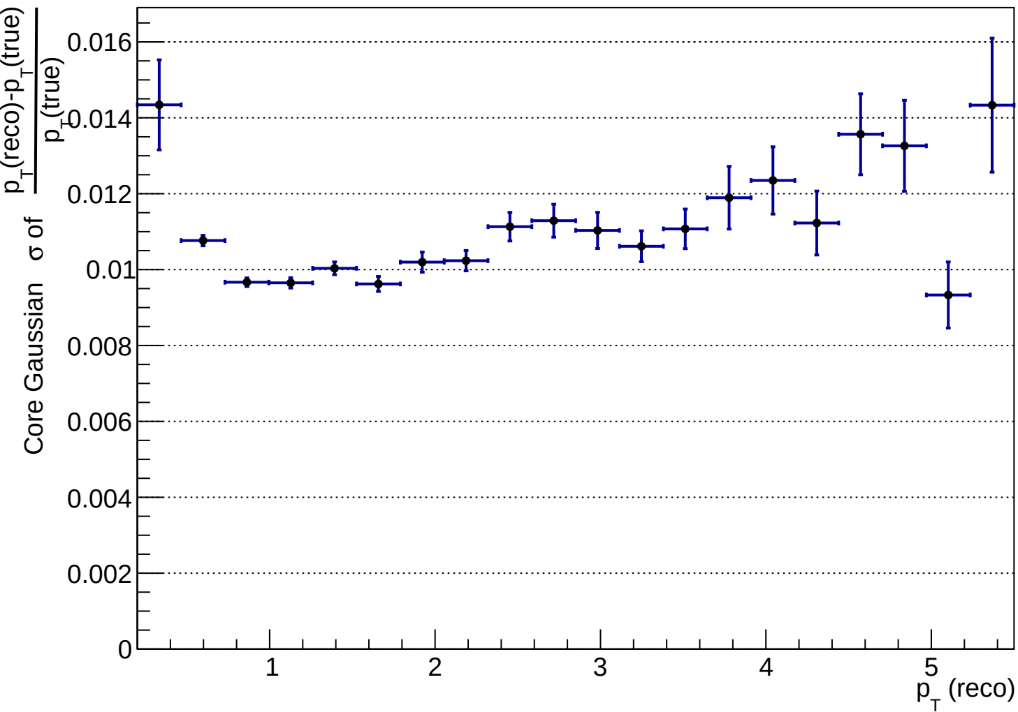
hptRes_vs_ptreco_K+
