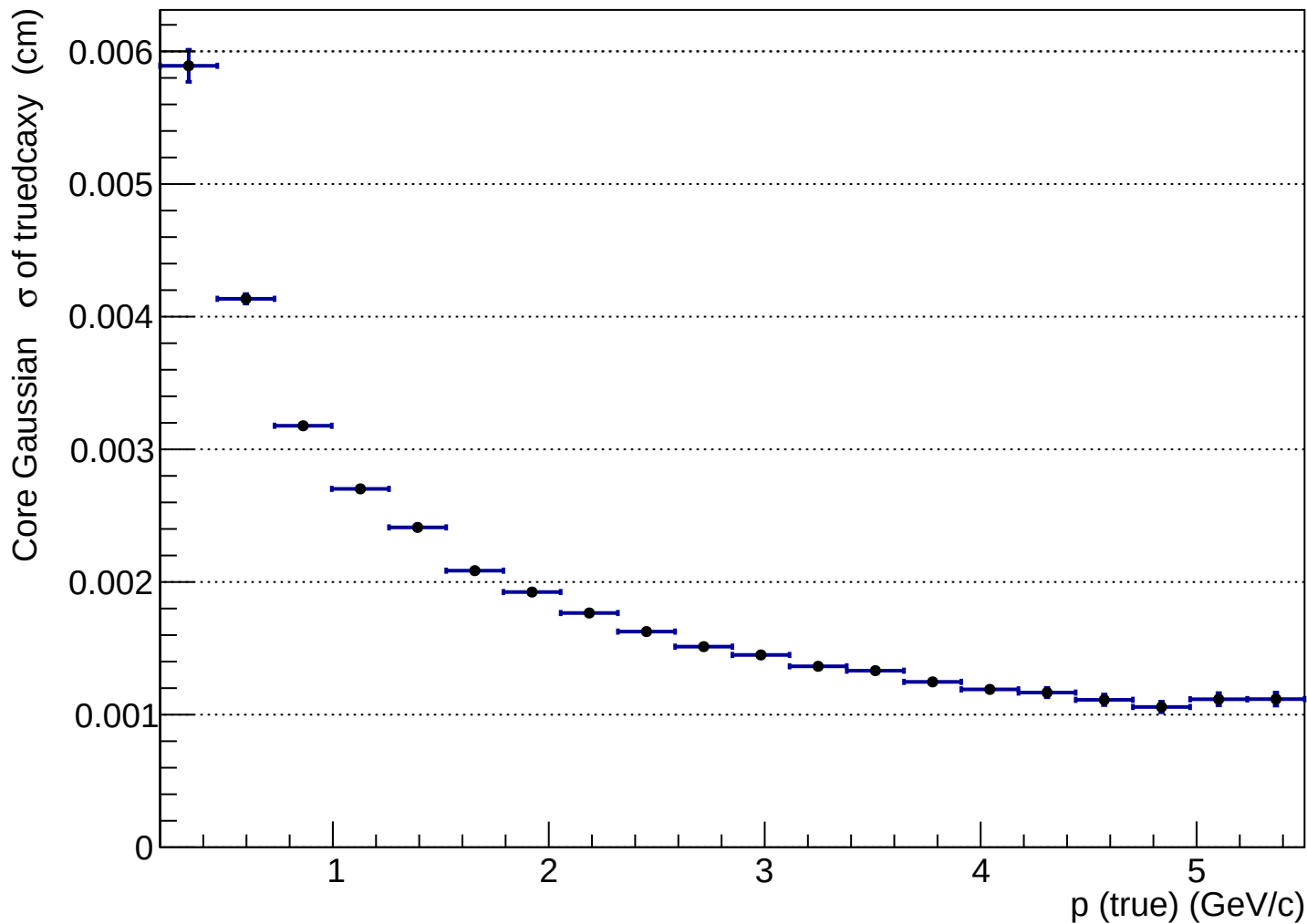
htruedcaxy_vs_ptrue_pi-
