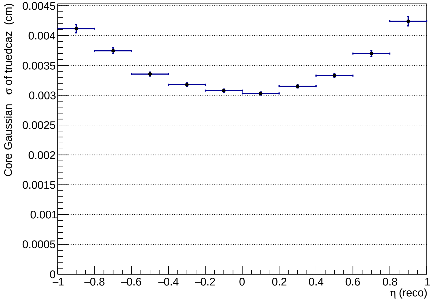
htruedcaz_vs_eta reco_pi+
