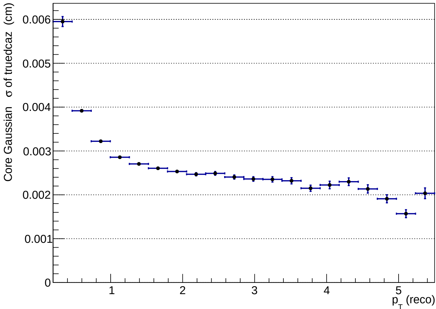
htruedcaz_vs_ptreco_pi-
