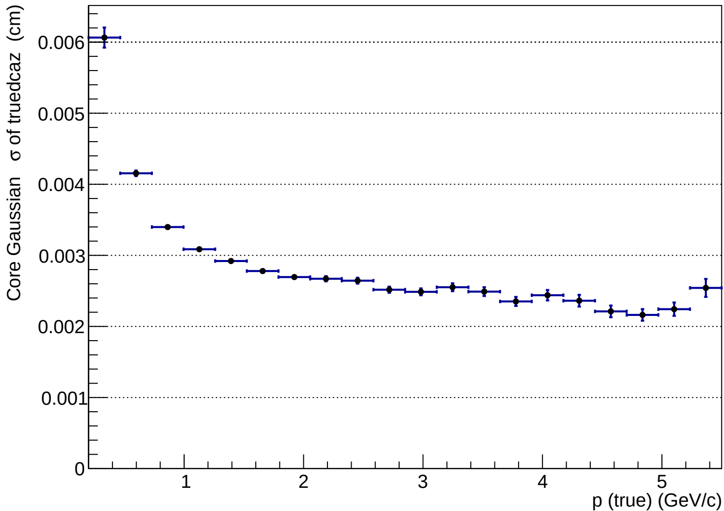
htruedcaz_vs_ptrue_pi-
