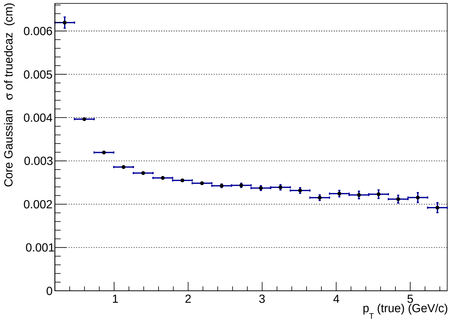
htruedcaz_vs_pttrue_pi+
