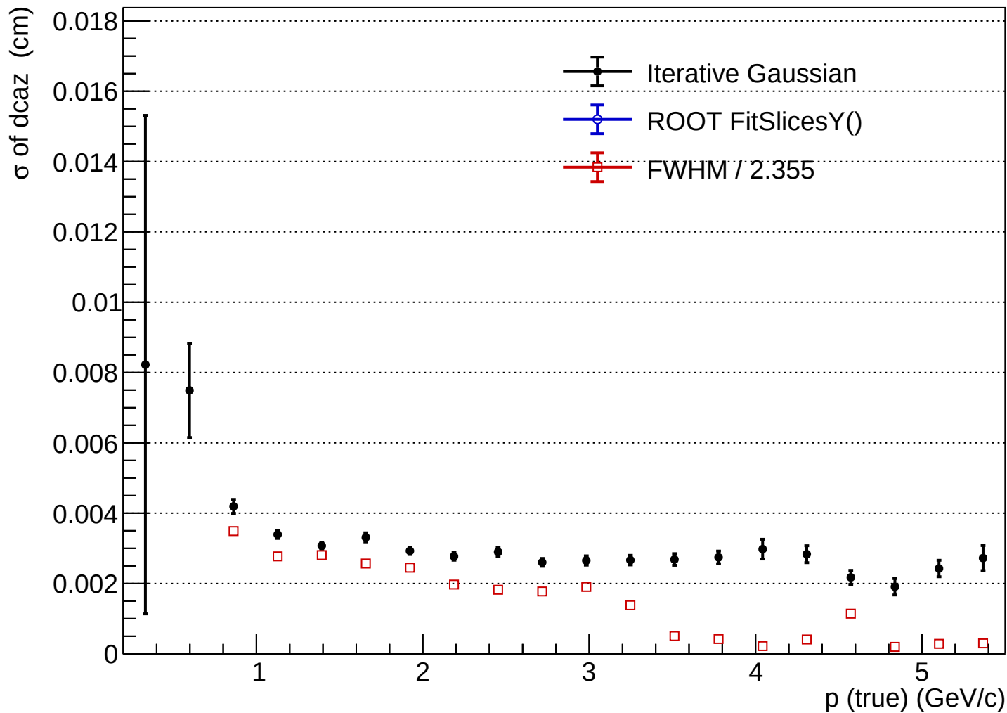
hdcaz_vs_ptrue_p
