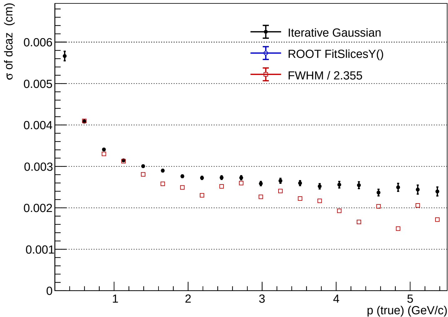
hdcaz_vs_ptrue_pi+
