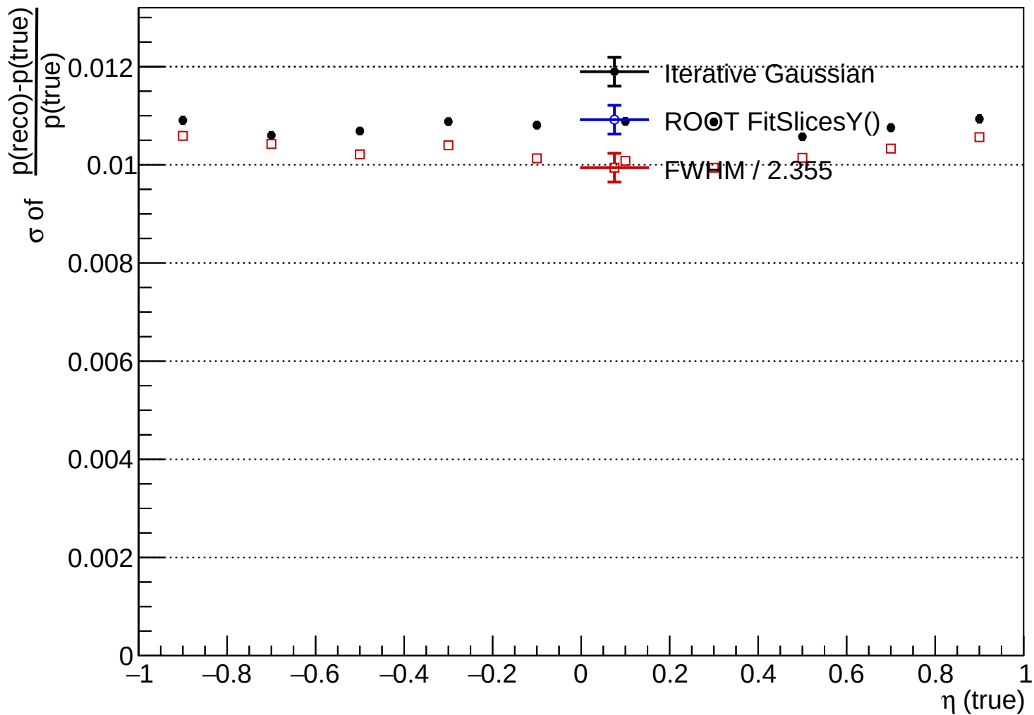
hpRes_vs_etatrue_pi-
