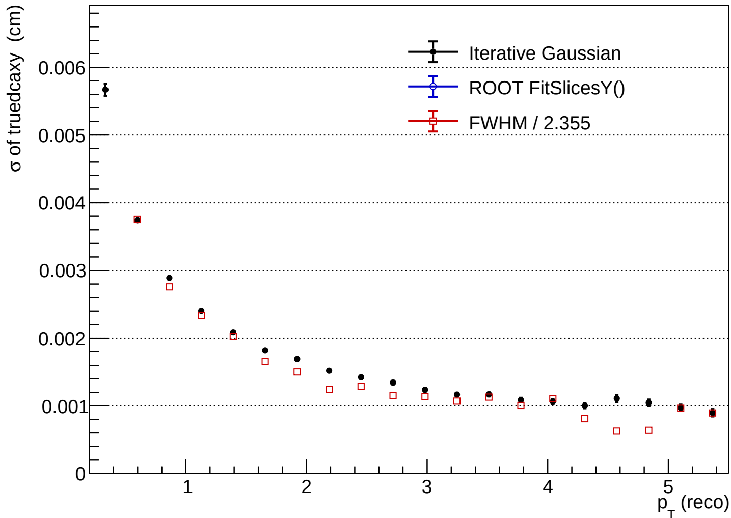
htruedcaxy_vs_ptreco_pi-
