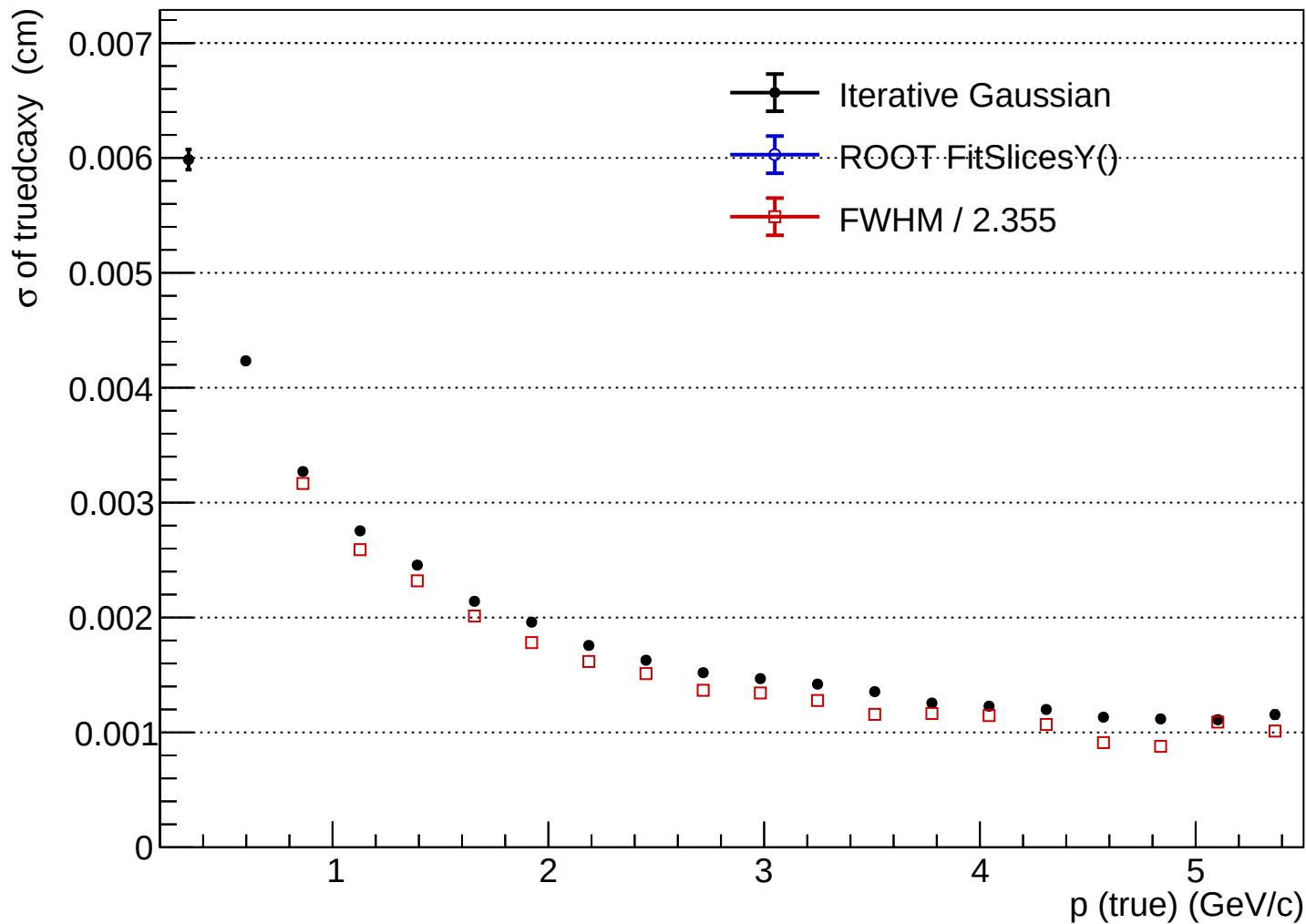
htruedcaxy_vs_ptrue
