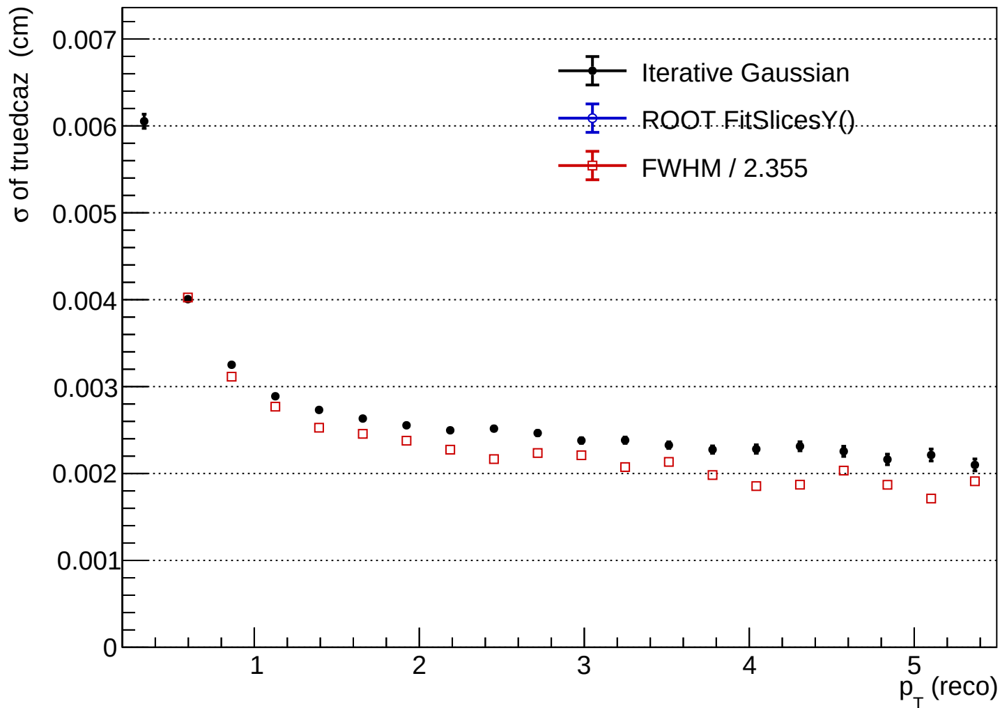
htruedcaz_vs_ptreco
