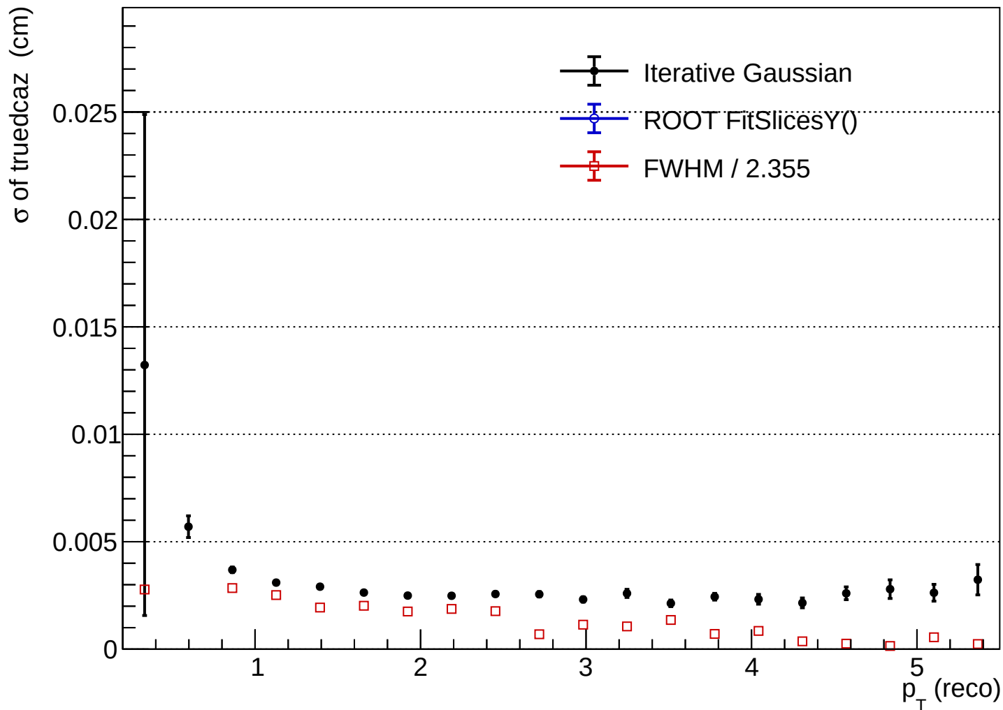
htruedcaz_vs_ptreco_p
