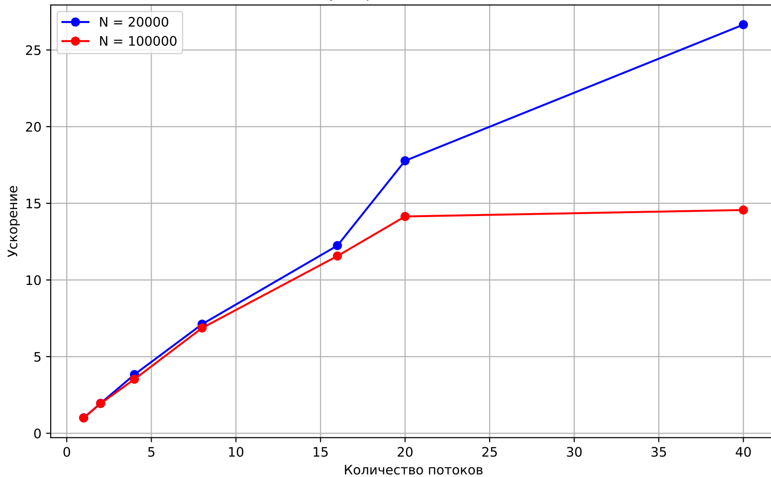
Зависимость ускорения от количества потоков
