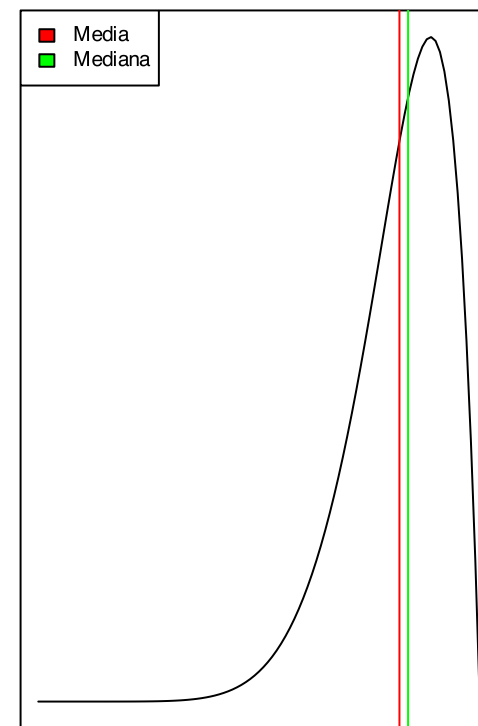
Asimmetria Negativa
