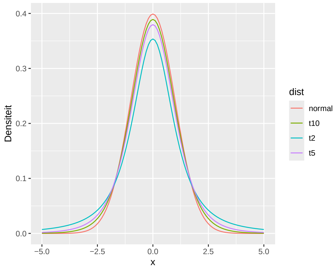
Figuur 6.7: Normale verdeling en t -verdeling met verschillende vrijheidsgraden.
