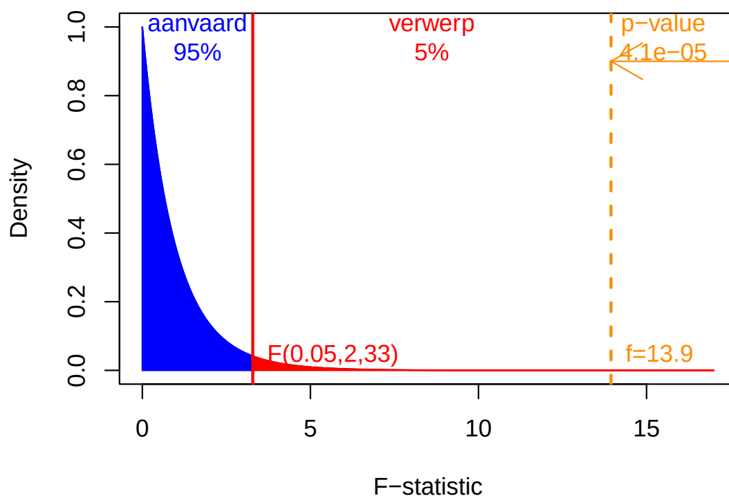
Figuur 8.5: Een F-verdeling met 2 vrijheidsgraden in de teller en 33 in de noemer. Het aanvaardingsgebied wordt weergegeven in blauw, de kritische waarde en de verwerpingsregio bij het \alpha = 5\% niveau in rood, en, de geobserveerde f-waarde en de p-waarde worden in oranje.
