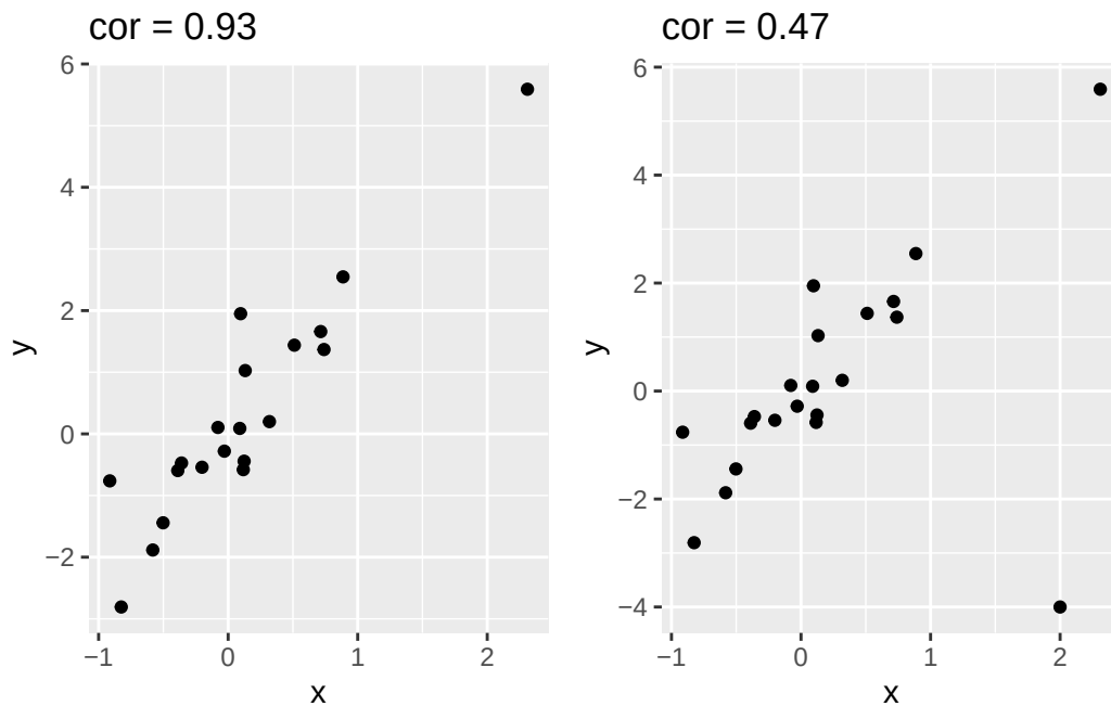
Figuur 5.8: Correlatie van gesimuleerde data met 1 outlier
