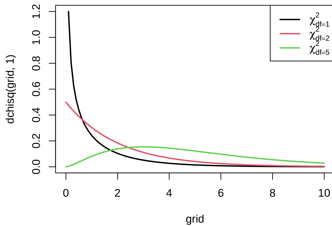
Figuur 10.5: Dichtheidsfuncties voor enkele Chi-kwadraat verdelingen
