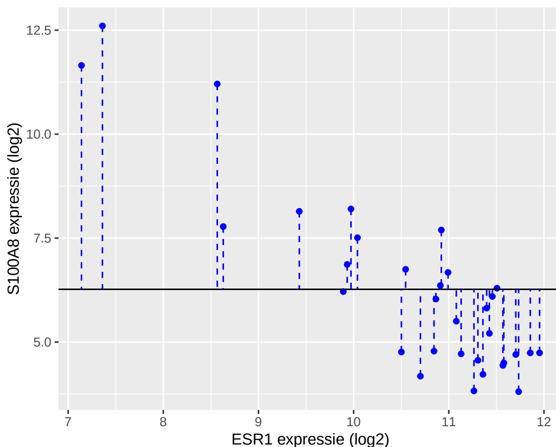
Figuur 7.12: Interpretatie van de totale kwadratensom ( SSTot ): de som van de kwadratische afwijkingen rond het steekproefgemiddelde.
