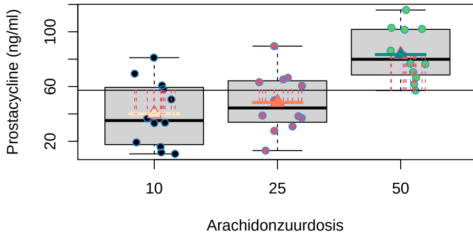
Figuur 8.3: Interpretatie van de kwadratensom van de behandeling (SST): de som van de kwadratische afwijkingen tussen de groepsgemiddelden ( \bar{Y}_j ) en het steekproefgemiddelde van de uitkomsten ( \bar{Y} )
