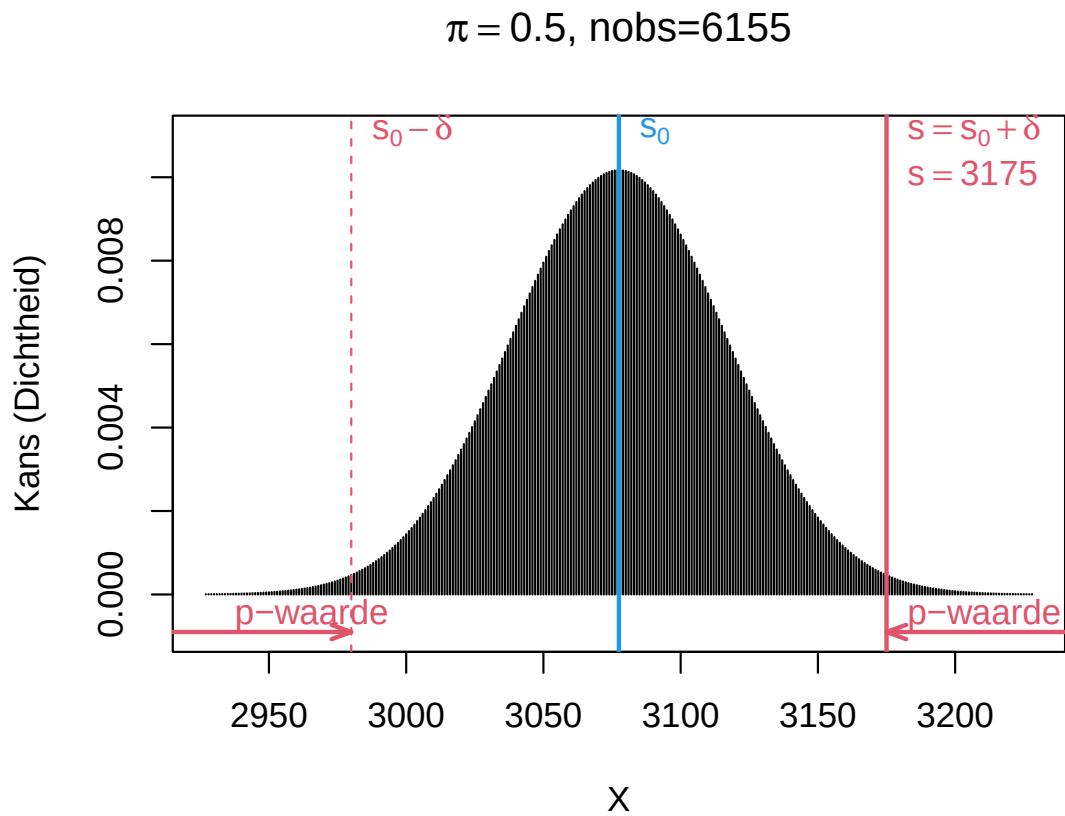
Figuur 10.3: Binomiale verdeling van het aantal jongens S onder H_0 : \pi = 0.5 ( n = 6155 ).
