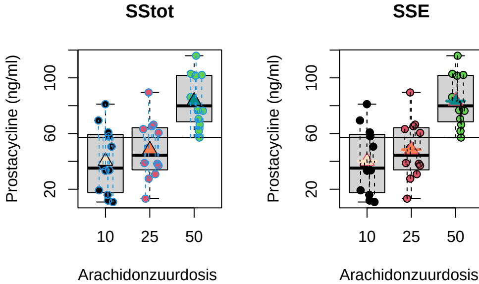
Figuur 8.4: Interpretatie van de totale kwadratensom ( SSTot , som van de kwadratische afwijkingen tussen de uitkomsten Y_i en het steekproefgemiddelde van de uitkomsten \bar{Y} , links) en van residuele kwadratensom ( SSE , som van de kwadratische afwijkingen tussen de uitkomsten Y_i en de groepsgemiddelden \bar{Y}_j , rechts)
