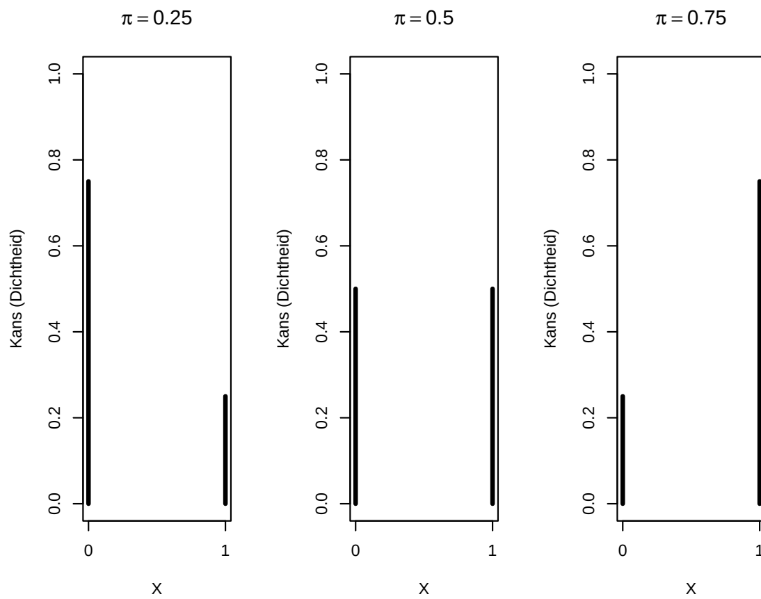
Figuur 10.1: Bernoulli verdelingen.
