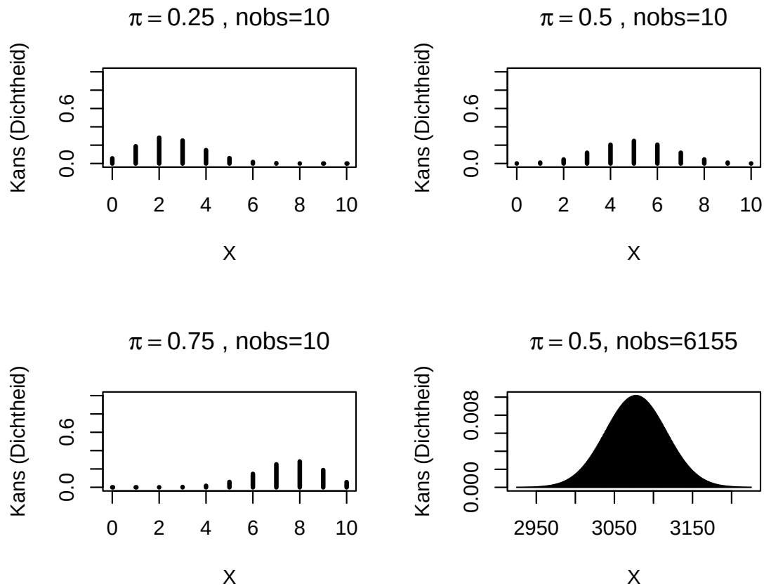
Figuur 10.2: Binomiale verdelingen.
