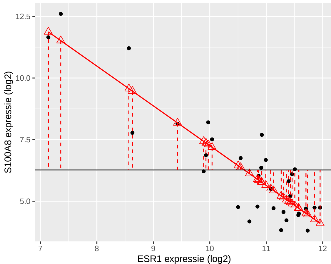
Figuur 7.13: Interpretatie van de kwadratensom van de regressie (SSR): de som van de kwadratische afwijkingen tussen de geschatte regressierechte en het steekproefgemiddelde van de uitkomsten.
