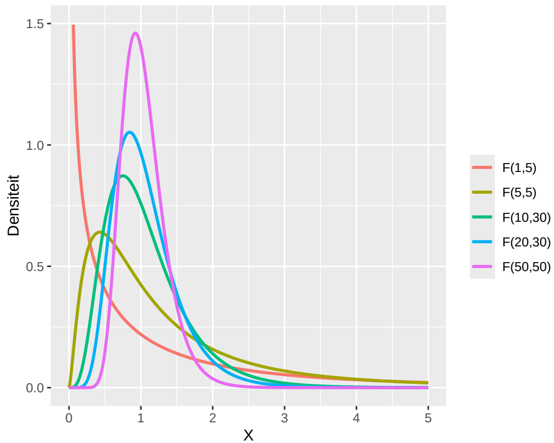
Figuur 8.6: Meerdere F-verdelingen met een verschillend aantal vrijheidsgraden in de teller en de noemer.
