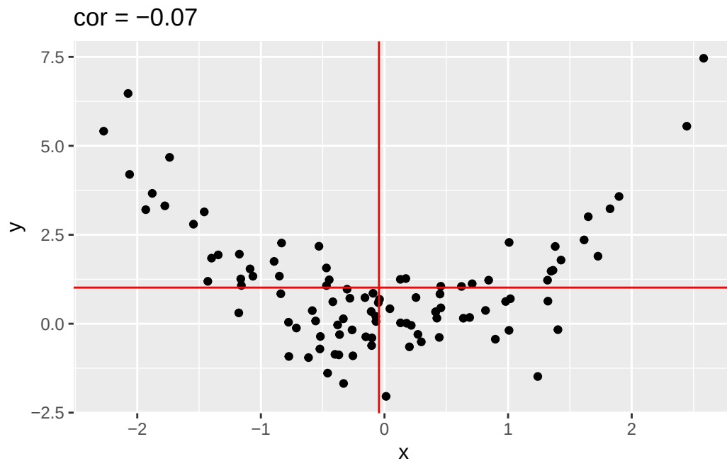
Figuur 5.9: Correlatie van gesimuleerde data met een kwadratisch verband. De data in de bovenste kwadranten compenseren elkaar als het ware alsook in de onderste kwadranten (ongeveer evenveel positieve en negatieve bijdragen door de data in de correlatie)
