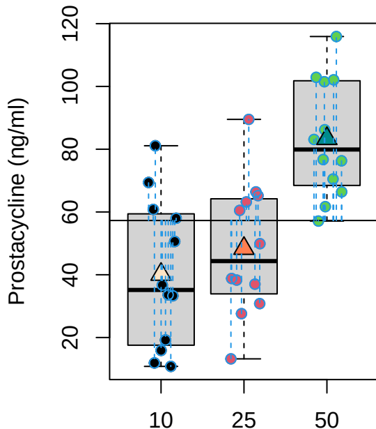
SStot
