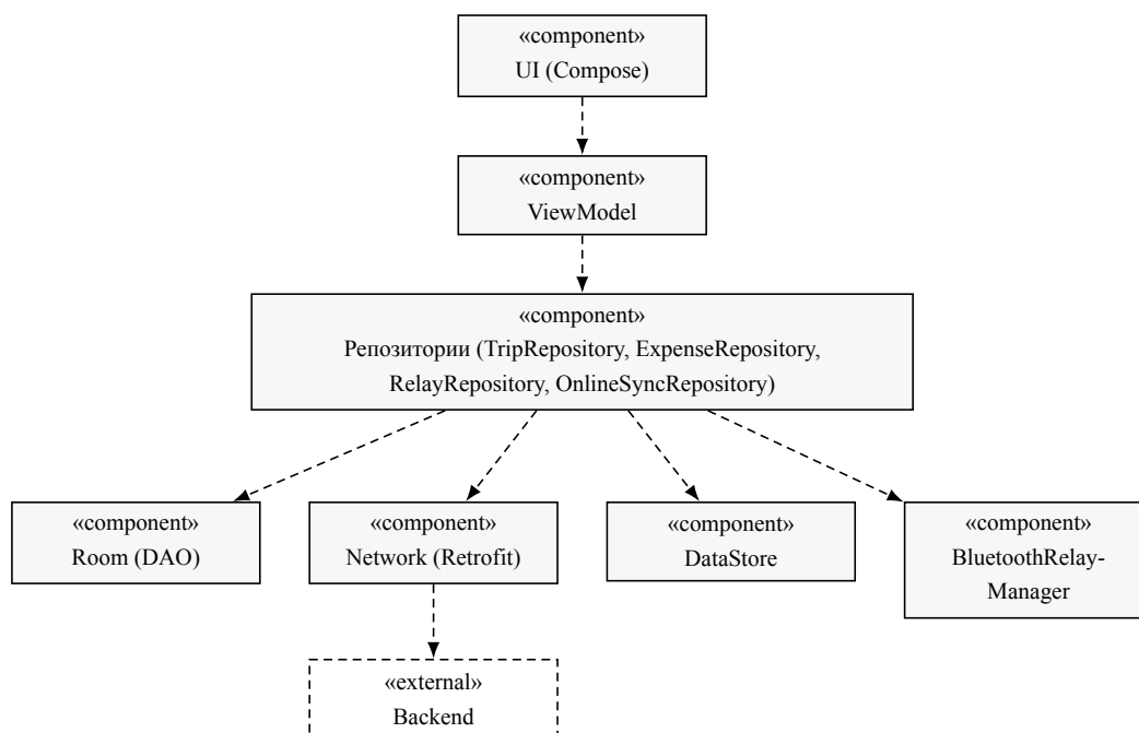
Рисунок 4. Схема компонентов клиента Triloo (зависимости показаны пунктиром)
