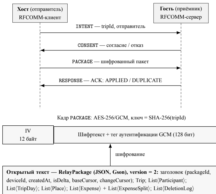
Рисунок 6. Протокол сессии Triloo Relay (вверху) и структура шифрованного пакета поездки (внизу)
