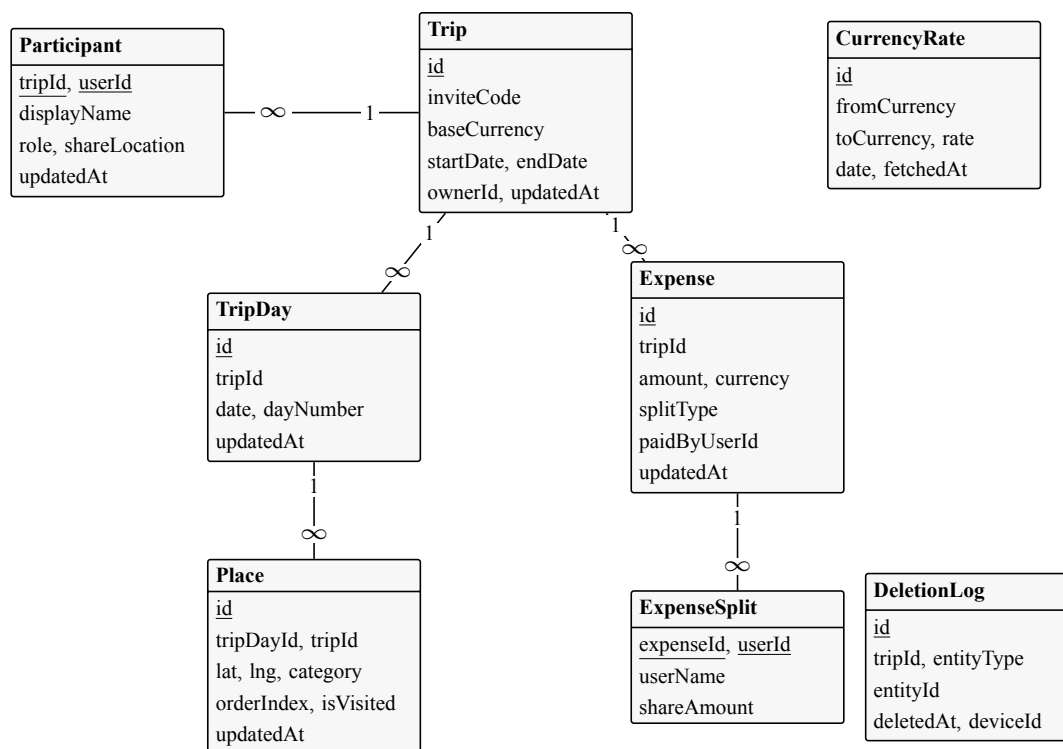
Рисунок 5. ER-схема доменной модели и локального хранилища Triloo ( подчёркнуты ключевые атрибуты)
