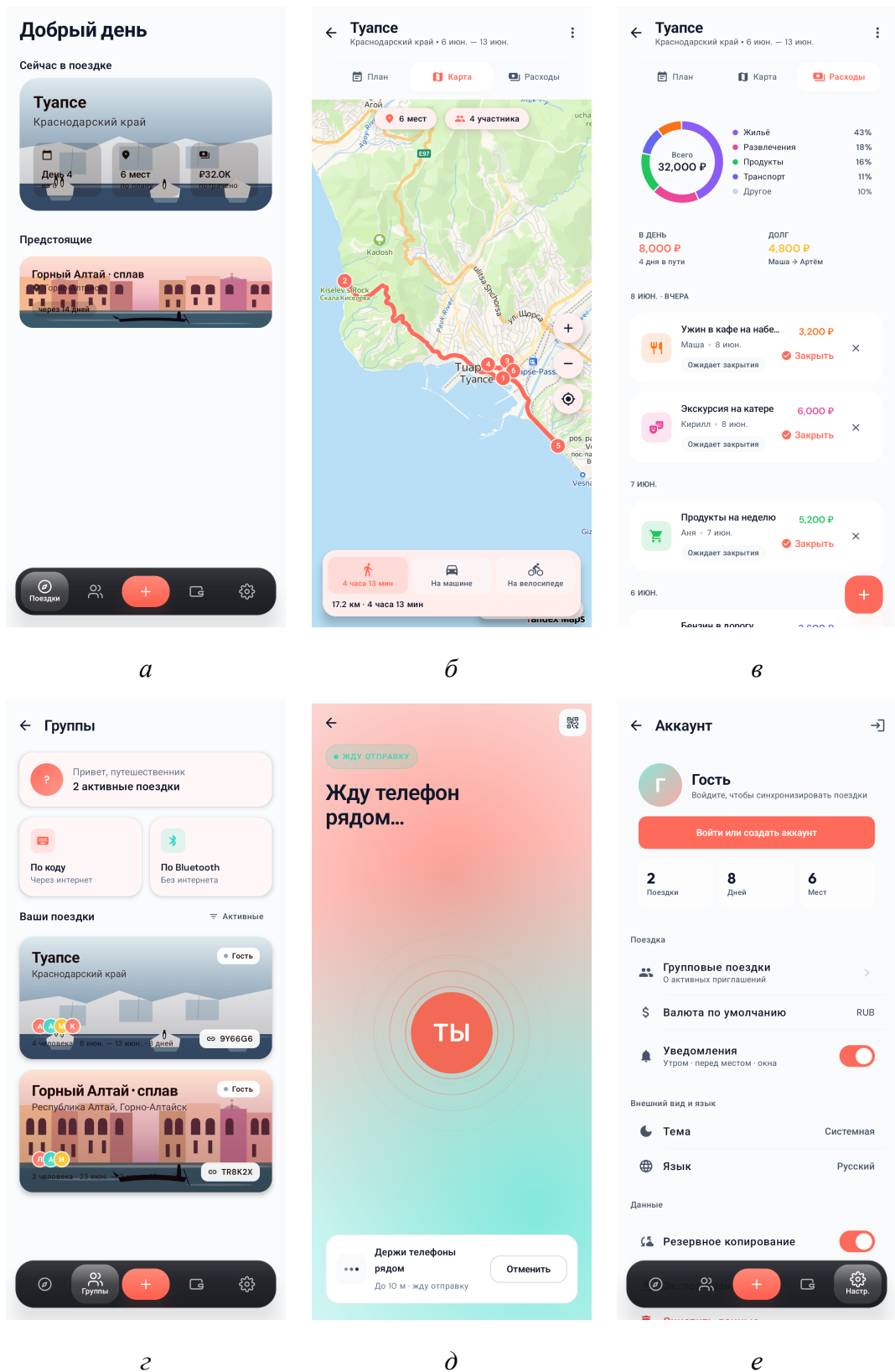
Рисунок 10. Основные экраны приложения Triloo: а — список поездок; б — карта поездки с участниками; в — учёт расходов; г — группы с инвайт-кодами и ролями; д — офлайн-обмен Triloo Relay; е — настройки
