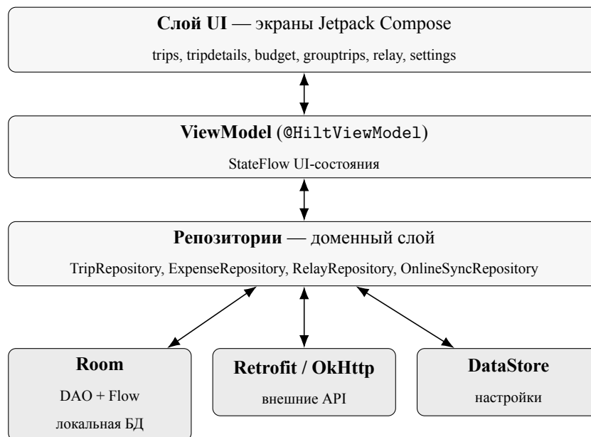
Рисунок 3. Многоуровневая offline-first-архитектура клиента Triloo
