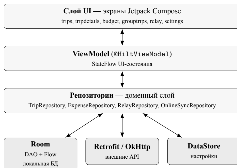
Рис. 1. Многоуровневая offline-first-архитектура клиента Triloo
