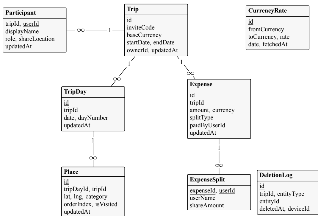
Рис. 2. ER-схема доменной модели и локального хранилища Triloo ( подчёркнуты ключевые атрибуты)
