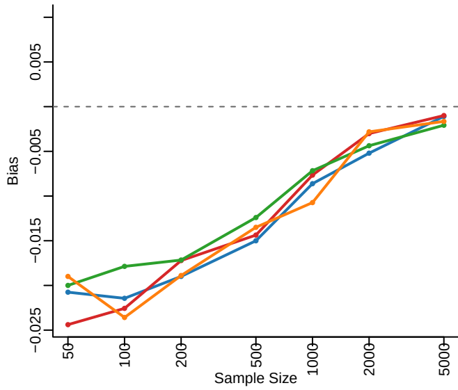
bmi: S=0.170
