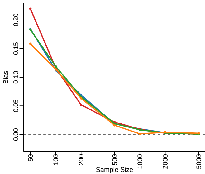
sex: S=0.068
