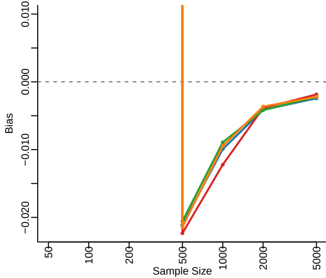
sex: S=0.000
