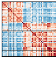
ENACT
