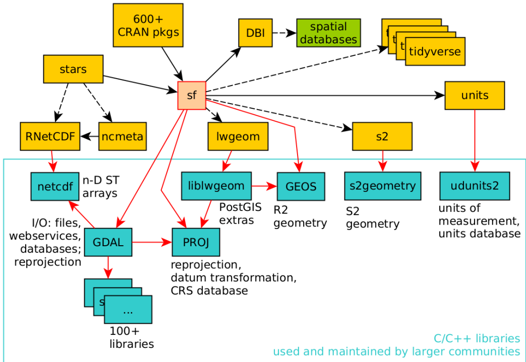
그림 2 sf 패키지와 의존성 - 화살표는 강한 의존성, 점선 화살표는 약한 의존성
