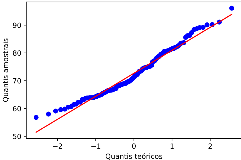
Q-Q plot (amostra)
