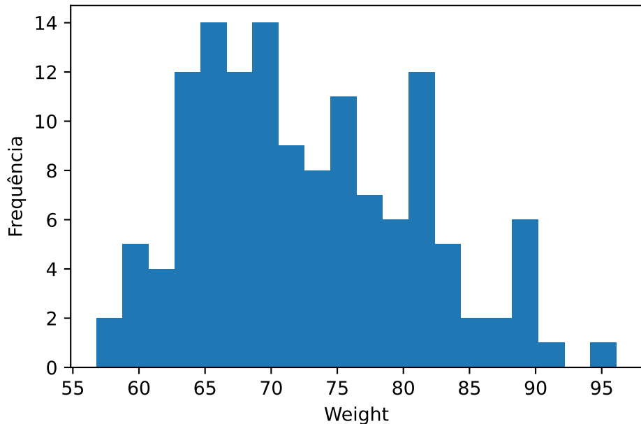
Histograma da variável weight
